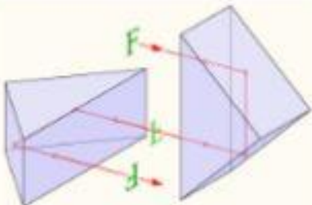
Pravoúhlý hranol
